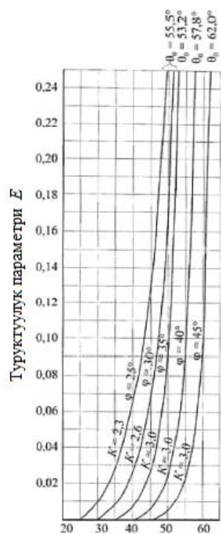
Горизонталдык жактан эңкейиш бурчу \theta , дар.
