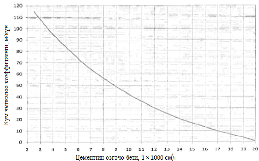
Т.1-сүрөт – Цемент эритмесинин өтүү жөндөмдүүлүгүнүн цементтин салыштырма бетине жана K_\phi карата графиги
