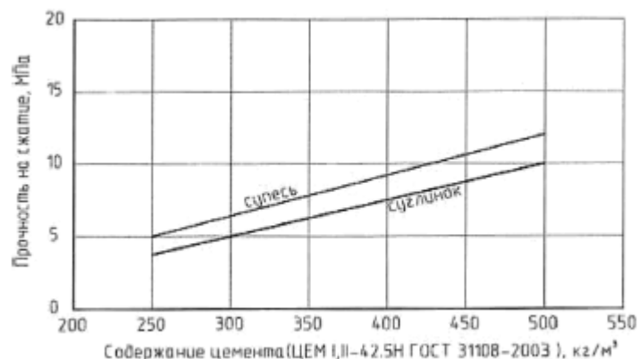
Рисунок Ф.3 – Зависимость прочности грунтоцемента от содержания цемента в 1 м³ ГЦЭ
