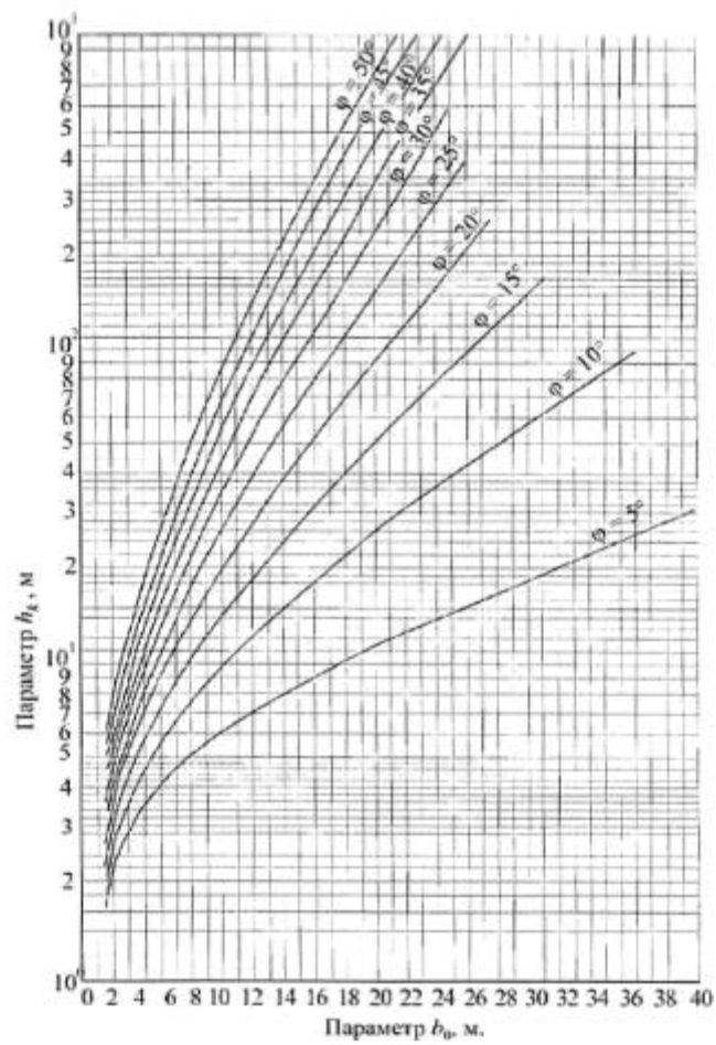
Рисунок В.6 – Графики для определения параметра b_0
