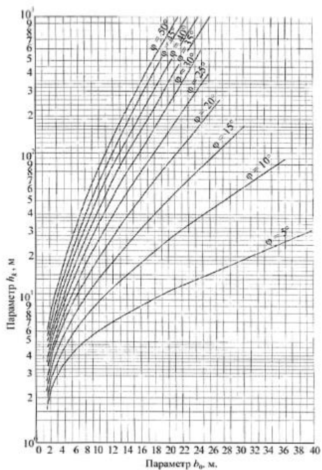
В.6-сүрөт – b_0 параметрин аныктоо үчүн графиктер
